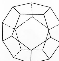
додекаедар тело са 12 страна
