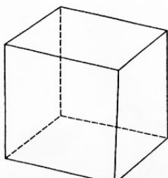
коцка или хексаедар тело са 6 страна
