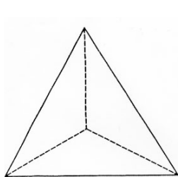
тетраедар тело са 4 стране
