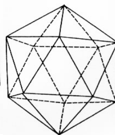
икосаедар тело са 20 страна
