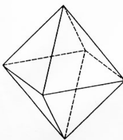
октаедар тело са 8 страна
